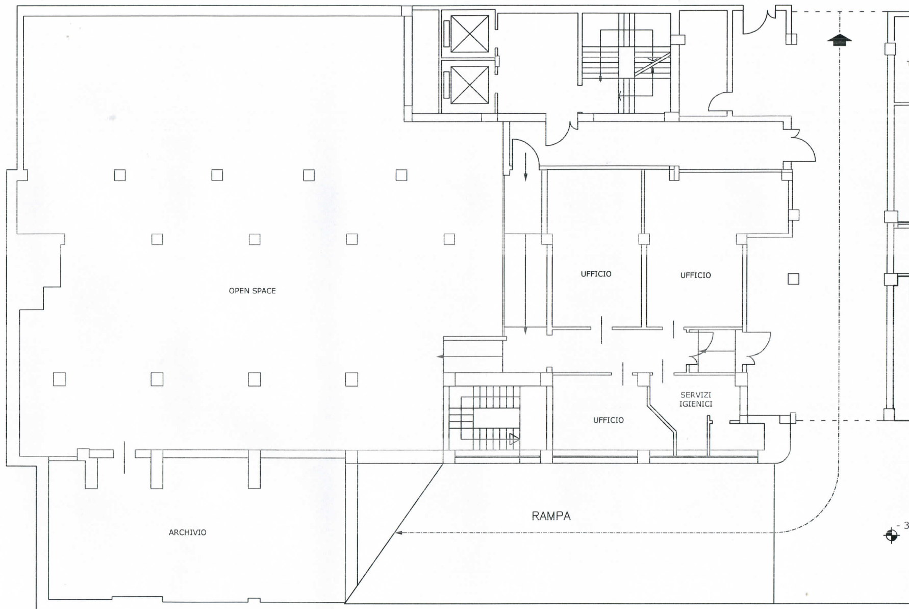
COLOMBO IMMOBILIARE 81 S.p.A. - Edificio di Via Cristoforo Colombo, 149 PLANIMETRIA PIANO 1° INTERRATO - Porzione da locare
